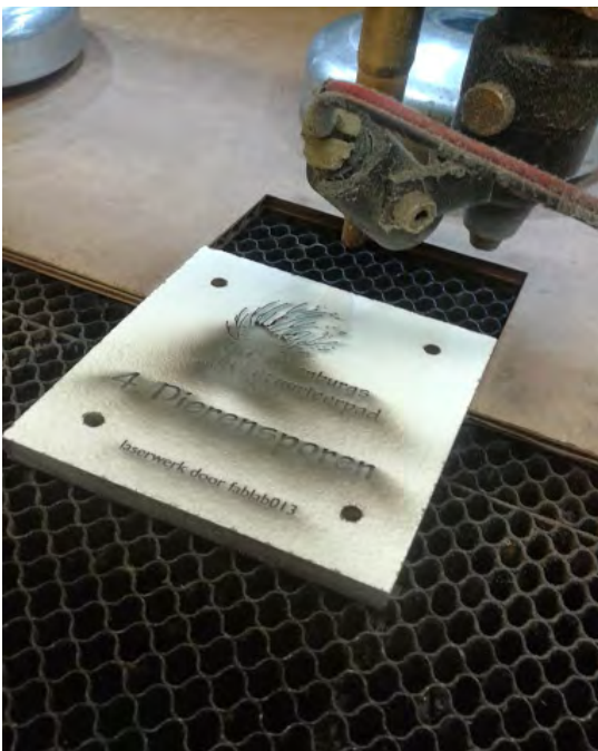
productie van bordjes d.m.v. lasertechnologie
